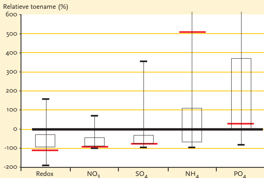
Fig. 4. Gemiddelde veranderingen in de waterbodem na verwijderen van isoetiden (rode lijn) en bij permanente inundatie (boxplots). Dit na 8 weken en in vergelijking met isoetidenrijke bodems respectievelijk droog gezette en weer vernatte bodems (zwarte nullijn). Resultaten van twee aparte proeven waarbij van 10 bodems wel en niet isoetiden zijn verwijderd en waarbij 41 bodems wel en niet tijdelijk zijn droog gezet.
