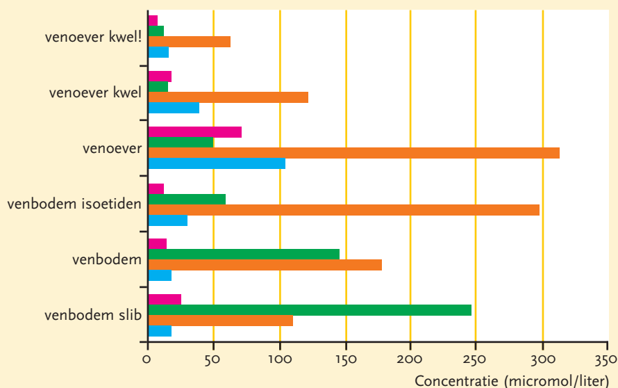
Fig. 3. Concentraties van vier ionen in het porievocht van zes typen standplaatsen in vennen; drie typen venbodem (32x slib, 40x venbodem, 20x isoetiden) en zeer ondiep grondwater uit drie typen venoeveren (25x oever, 11x kwel, 12x kwel!).
