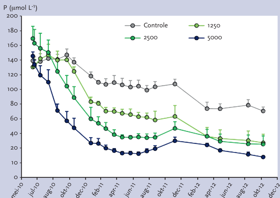
Fig. 3. Verbrakkingsexperiment in het IJperveld. Effecten van verschillende zoutconcentraties in de waterlaag (controle en respectievelijk 1250, 2500 en 5000 mg Cl.L⁻¹) op de fosforconcentratie van het bodemwater (naar van Dijk et al., 2013).
