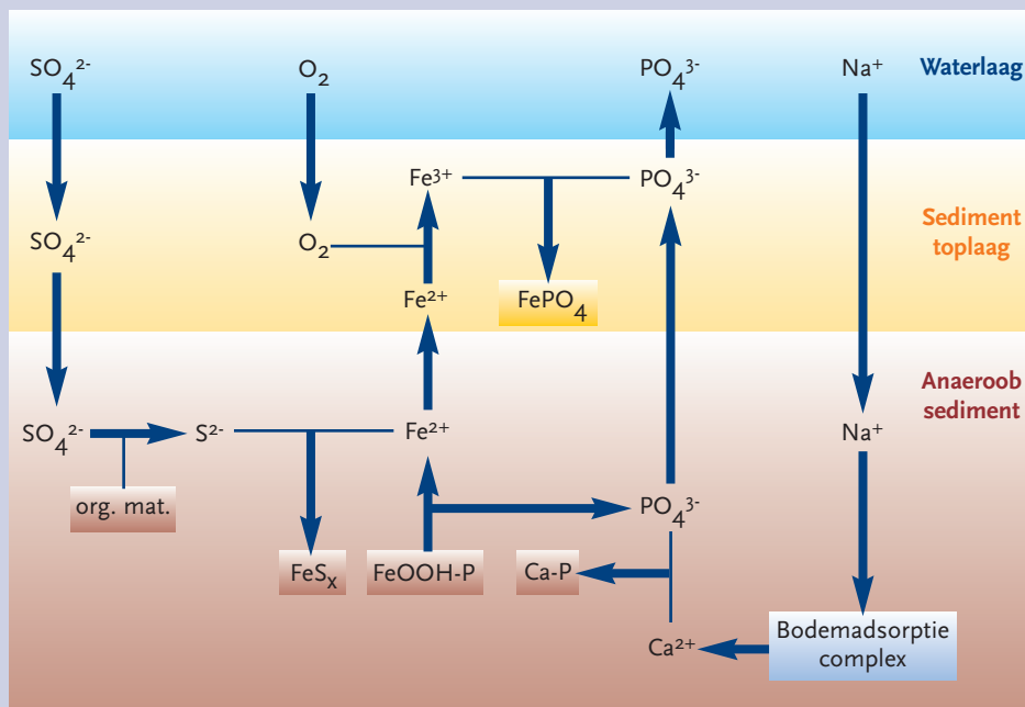
Fig. 4. Schematische voorstelling van de interacties tussen ijzer, fosfor, zwavel, natrium en calcium in de onderwaterbodem van veenweidegebieden en de effecten van verbrakking.
