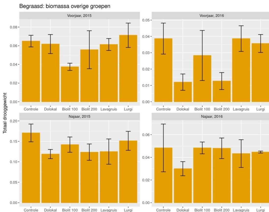
Figuur 9.18. Gemiddelde biomassa van overige ongewervelde groepen in sleepnetmonsters in de verschillende behandelingen van enkel de begraasde proefvlakken ( n=3 ), per bemonsteringsmoment (voorjaar/najaar, 2015/2016). Let op de verschillen in schaal van de y-as per grafiek. Error bars geven \pm 1 S.E. weer.
