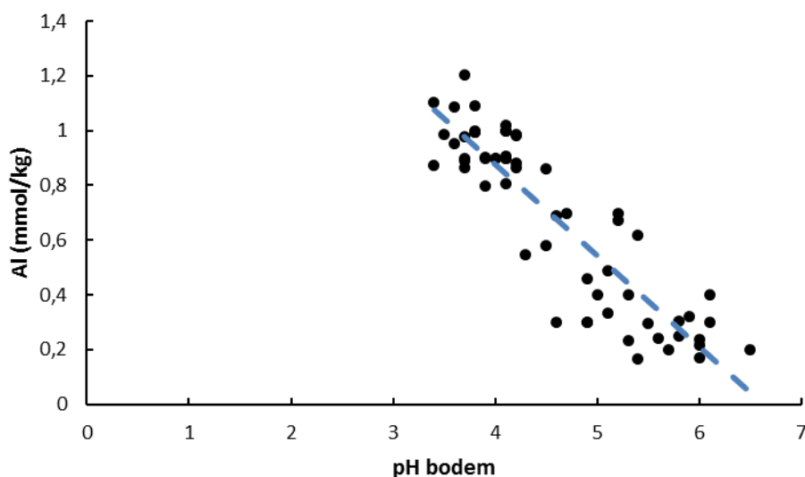
Figuur 8.4. Al-gehalten (in mmol/kg drooggewicht) in bladeren van Veldzuring bij verschillende pH-waarden van de bodem.
