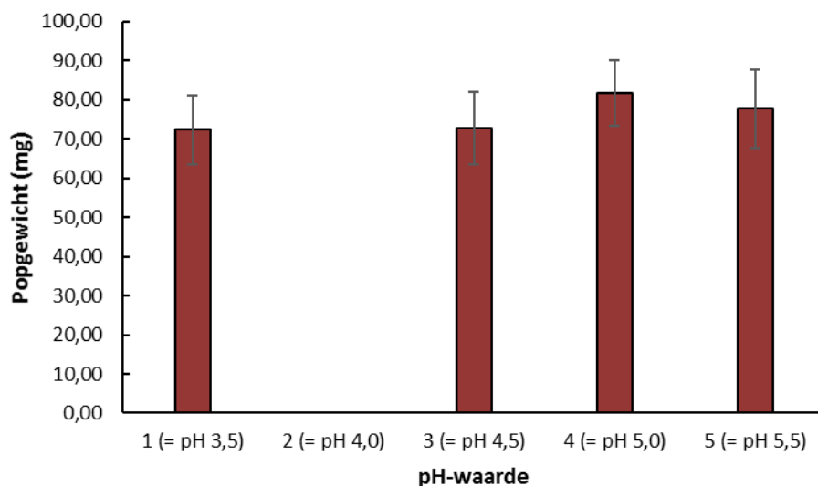
Figuur 8.7. Popgewicht (mg) van Kleine vuurvlinders (2e generatie) opgekweekt op Veldzuring bij verschillende pH-waarden. N.B. De dieren van pH-groep 4.0 uit de eerste generatie bleken allen mannelijk, er is hier geen 2e generatie.
