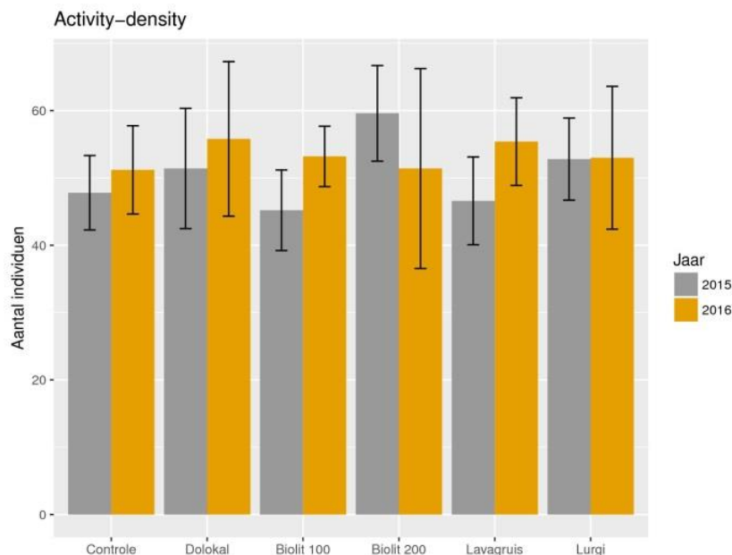
Figuur 9.4. Gemiddelde activity-density van alle loopkevers in de verschillende behandelingen, uitgesplitst over beide bemonsteringsjaren. Error bars geven \pm 1 S.E. weer. *: significant verschillend ten opzichte van controle.
