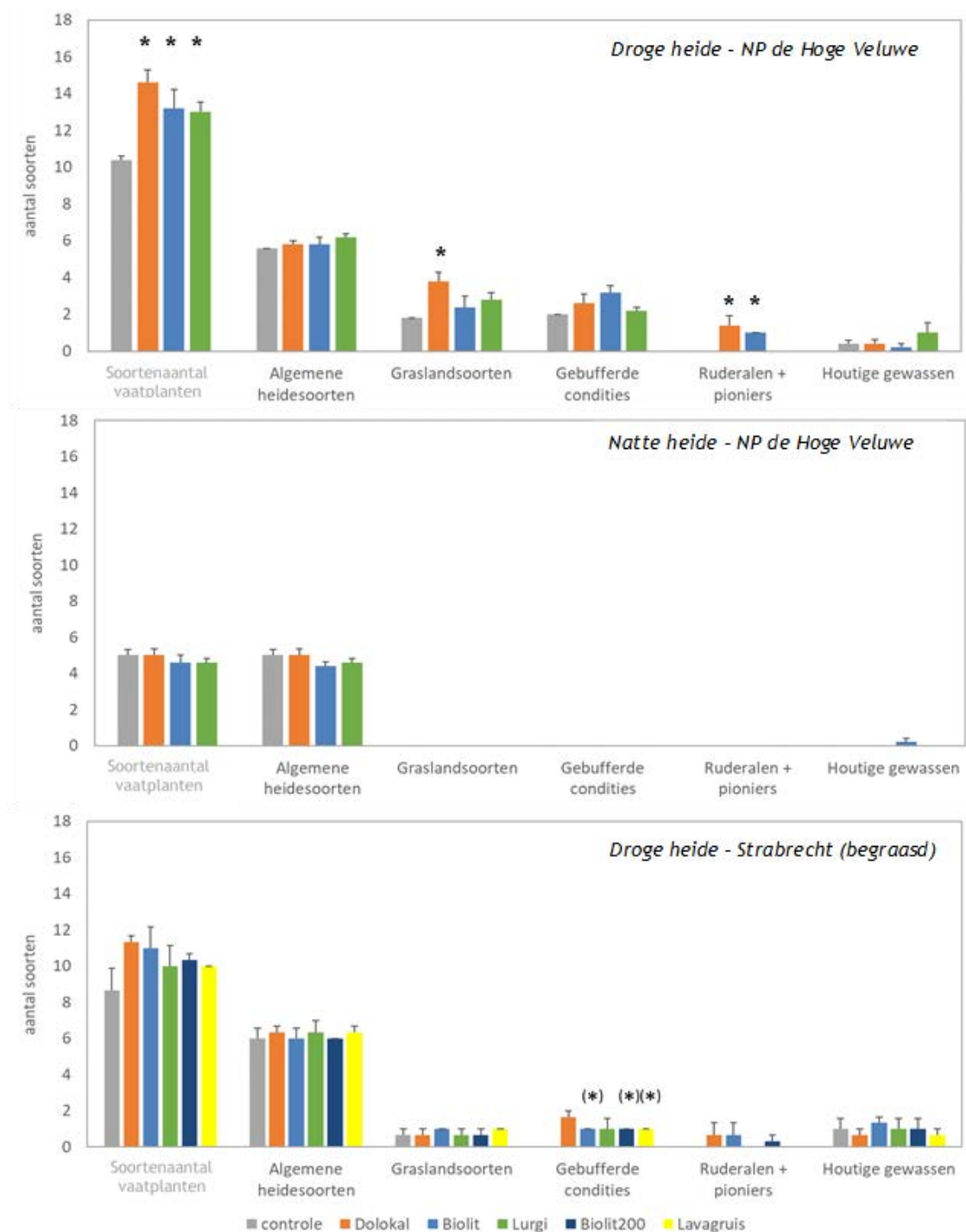
Figuur 7.6. Totaal aantal soorten vaatplanten en de verdeling over verschillende soortgroepen in 2017 ( \bar{x} \pm \text{standaardfout} ).
