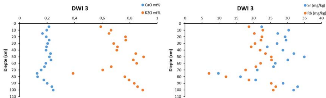
Figuur 4.12. Kalium laat verweringsprofiel op overstoven E-horizont zien (links) en Sr en Rb tonen stuifzand op E-horizont van onderliggend dekzand (rechts).
