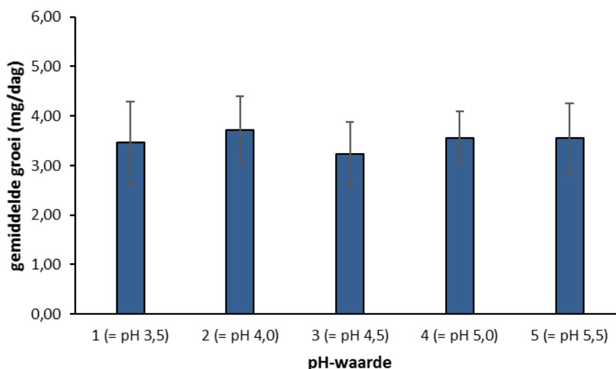
Figuur 8.9. De gemiddelde groei van de rupsen van Kleine vuurvliinder per dag in het experiment met Biolit als bufferstof.
