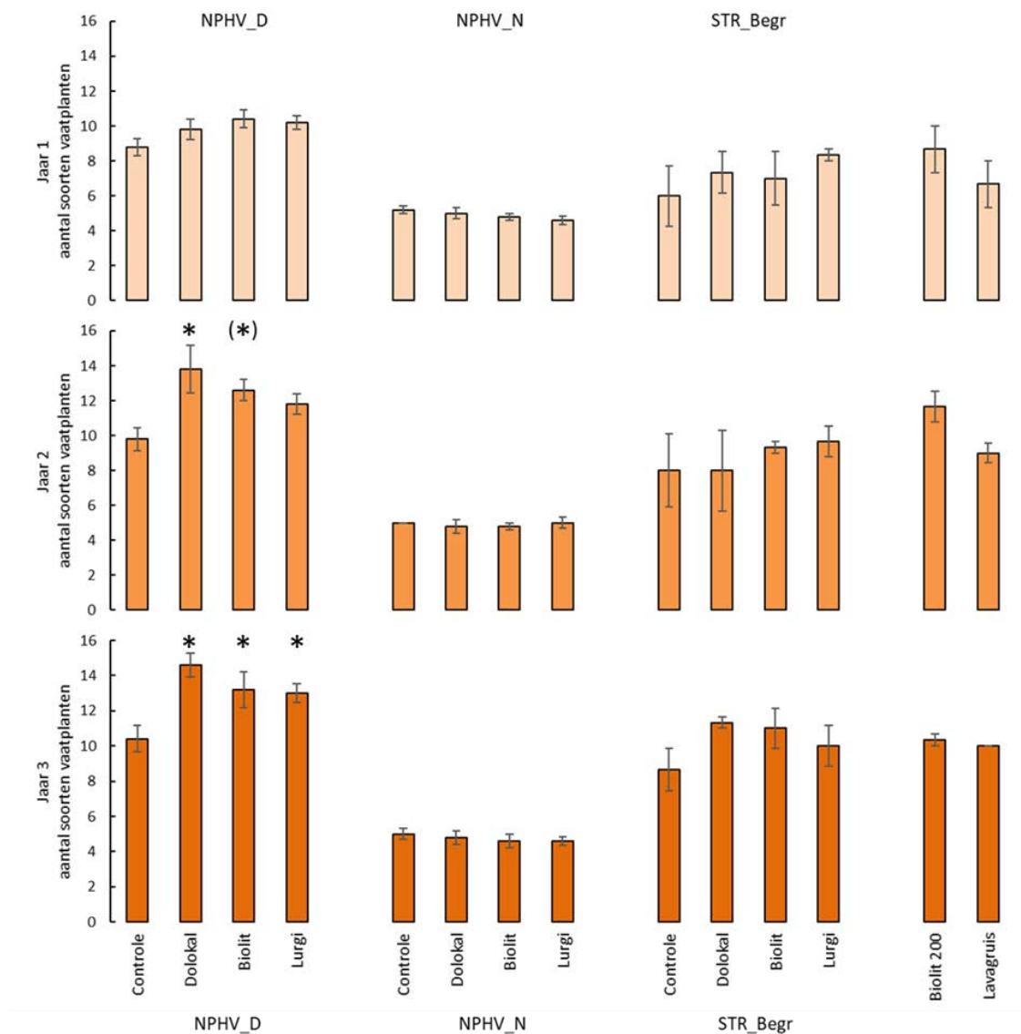
Figuur. 7.4. Aantal soorten vaatplanten per behandeling ( \bar{x} \pm \text{standaardfout} ) in 2015, 2016 en 2017. Biolit 200 en lavagruis zijn alleen toegepast op de Strabrechtse heide. * = significant verschil ( p < 0,05 ), (*) = trend ( 0,10 < p < 0,05 ).
