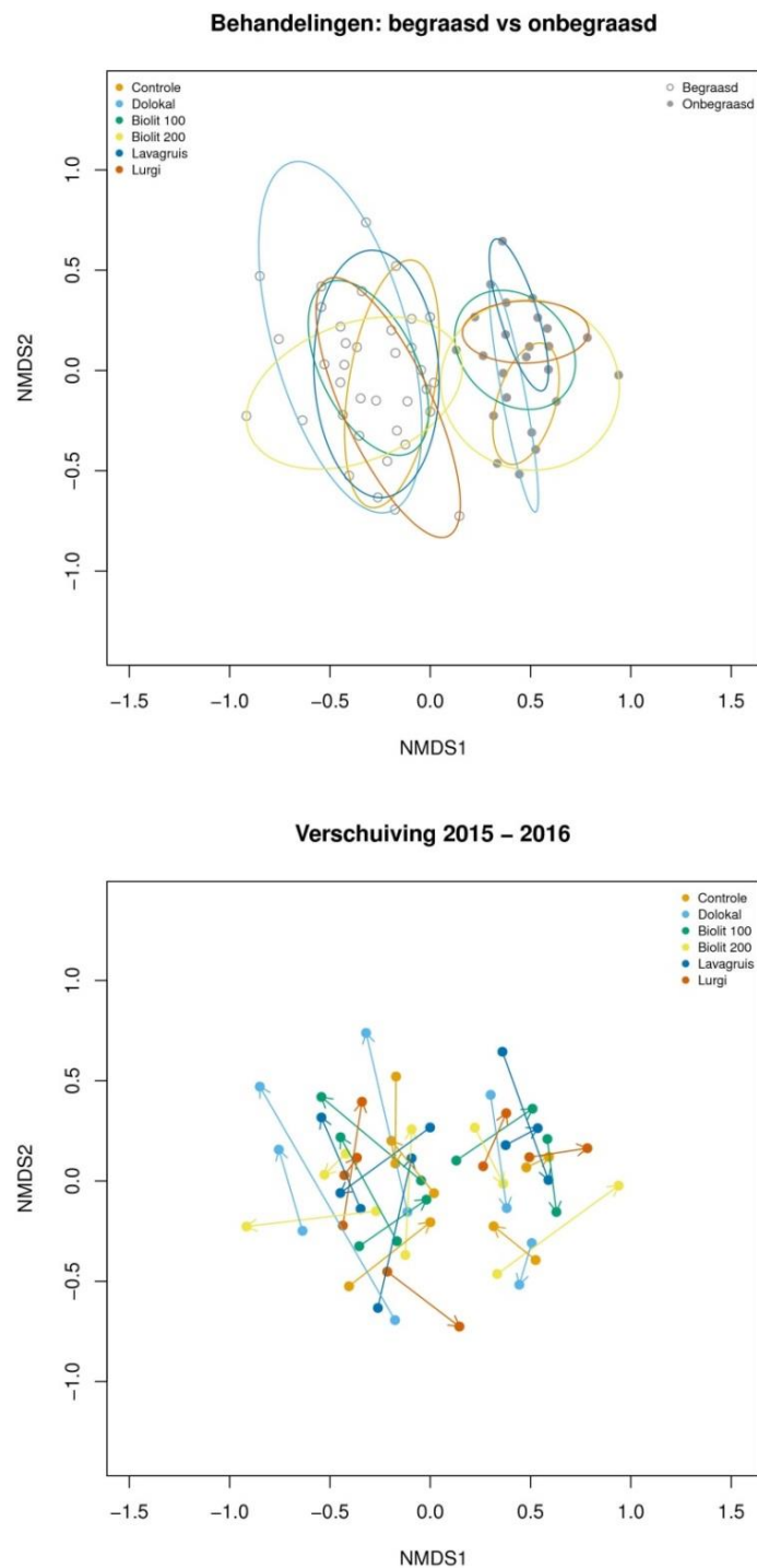
Figuur 9.2. NMDS plot van de loopkevervangsten uit 2015 en 2016 van alle onderzoeksplots. Boven: plaatsing van de monsterpunten in het ordinatiediagram, uitgesplitst over proefvlakken die in het begraasde deel gelegen zijn en proefvlakken die buiten de begrazingseenheid gelegen zijn. Ellipsen geven de plaatsingsrange van de verschillende behandelingen weer. Onder: verschuivingen in het ordinatiediagram van verschillende monsterpunten tussen 2015 en 2016. Pijlen geven de verschuiving weer van 2015 naar 2016. Kleuren van de pijlen en ellipsen corresponderen met de verschillende behandelingen (zie legenda).
