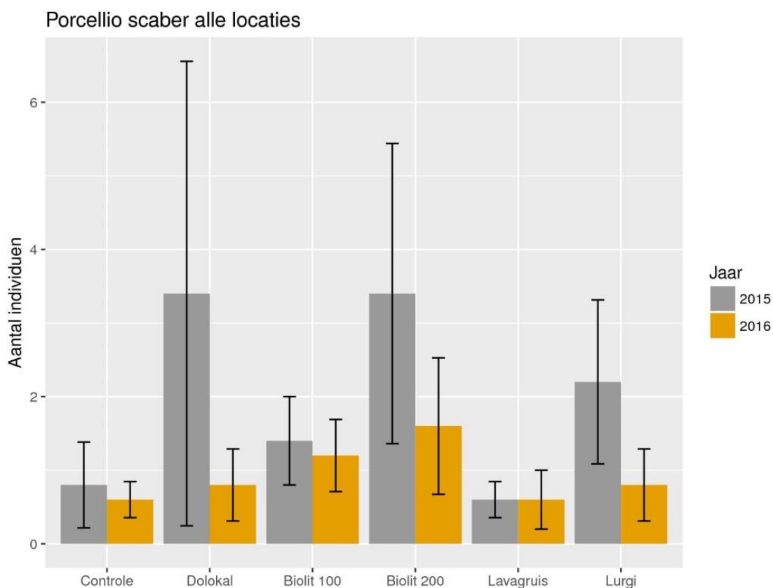
Figuur B6.10. Aantal bemonsterde individuen van Porcellio scaber in de verschillende behandelingen van alle proefvlakken, uitgesplitst over beide bemonsteringsjaren. Error bars geven \pm 1 S.E. weer. N.B. In de onbegraasde locaties ( n=2 ) is P. scaber in geen van beide onderzoeksjaren aangetroffen, waardoor de spreiding in de data (S.E. bars) sterk toeneemt. Figure B6.10. Mean number of trapped Porcellio scaber individuals in different treatments in all blocks ( n=5 ), in the different treatments per sampling year. In ungrazed blocks ( n=2 ), no individuals were found in either sampling year, resulting in a strong increase in S.E. bars. Error bars indicate \pm 1 S.E.
