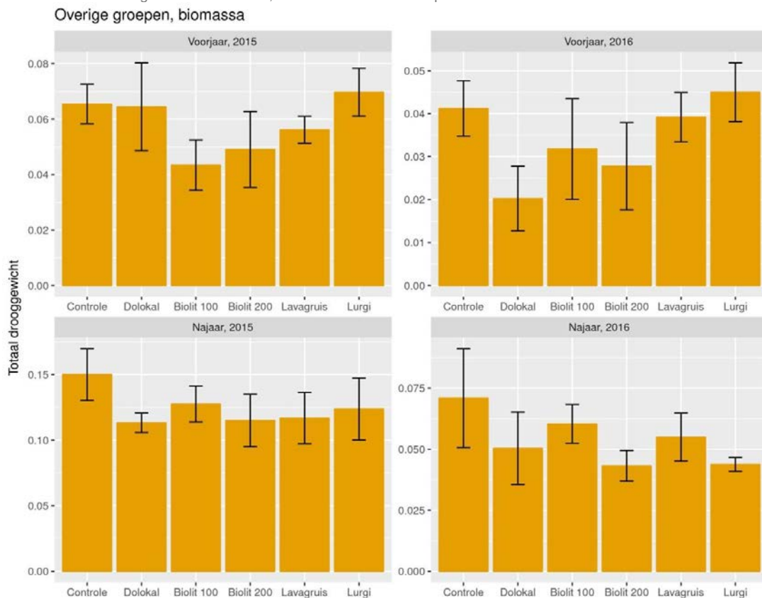
Figuur 9.16. Gemiddelde biomassa van overige ongewervelde groepen in sleepnetmonsters in de verschillende behandelingen (n=5), per bemonsteringsmoment (voorjaar/najaar, 2015/2016). Let op de verschillen in schaal van de y-as per grafiek. Error bars geven \pm 1 S.E. weer.
