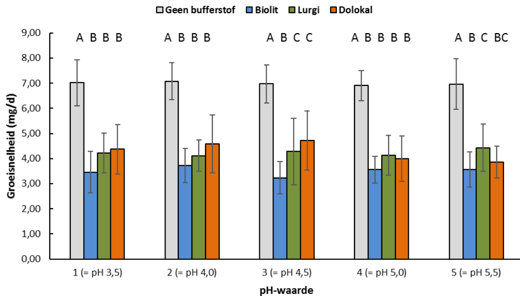
Figuur 8.13. Vergelijking van de dagelijkse groeisnelheid van Kleine vuurvliinder in de experimenten met de vijf verschillende pH groepen, zonder en met bufferen met resp. Biolit, Lurgi en Dolokal als toegevoegde bufferstof. Verschillende letters geven significante verschillen weer tussen groepen Figure 8.13. Average growth per day of Lycaena phlaeas caterpillars per treatment. Different letters represent significant different groups.
