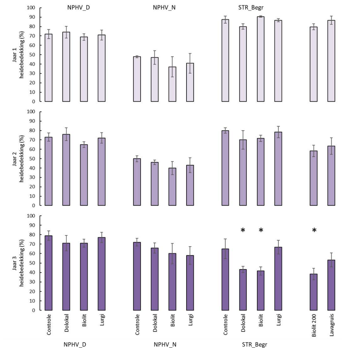
Figuur 7.2. Ontwikkeling van de bedekking van heidesoorten ( \bar{x} \pm standaardfout) in de drie jaren na de toediening van de verschillende behandelingen. Biolit 200 en lavagruis zijn alleen toegepast op de Strabrechtse heide. * = significant verschil ten opzichte van controle ( p < 0,05 ), (*) = 0,10 < p < 0,05 .
