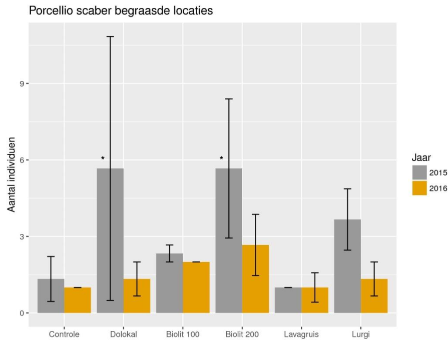
Figuur 9.14. Gemiddeld aantal bemonsterde individuen van Porcellio scaber in de verschillende behandelingen van enkel de begraasde proefvlakken (n=3), uitgesplitst over beide bemonsteringsjaren. Error bars geven \pm 1 S.E. weer. *: significant verschillend ten opzichte van controle.
