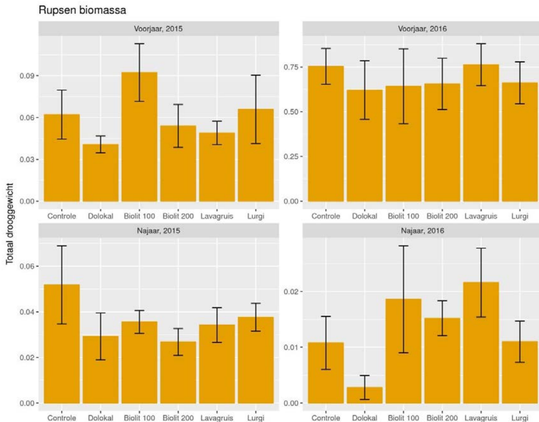
Figuur 9.15. Gemiddelde biomassa van rupsen in sleepnetmonsters in de verschillende behandelingen (n=5), per bemonsteringsmoment (voorjaar/najaar, 2015/2016). Let op de verschillen in schaal van de y-as per grafiek. Error bars geven \pm 1 S.E. weer.
