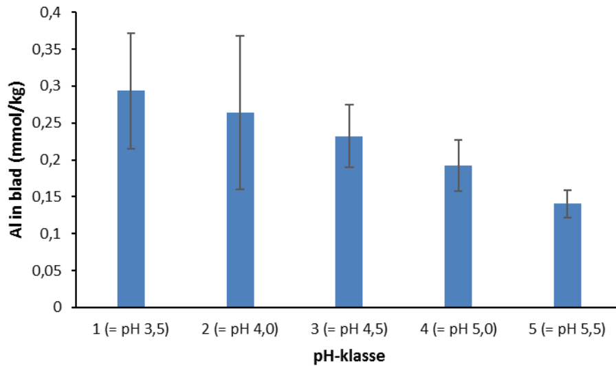
Figuur 8.5. Al-gehalten in mmol/kg in bladeren van Veldzuring bij de verschillende pH-classes in de experimenten (1= pH 3,5, 2= pH 4,0, 3= pH 4,5, 4= pH 5,0 en 5= pH 5,5).
