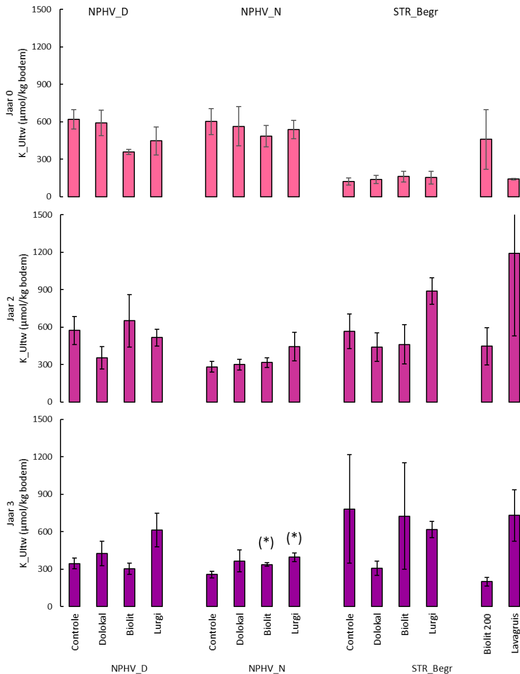
Figuur 5.4. Uitwisselbare concentratie kalium ( \bar{x} \pm standaard fout, in \mu\text{mol/kg} bodem) in de nulmeting (jaar 0), na twee en na drie effectjaren in de droge proef in het NP de Hoge Veluwe (NPHV_D, links, n=5 ), de natte proeflocatie in het NP De Hoge Veluwe (NPHV_N, midden, n=5 ) en in de begraasde proefvlakken in de droge heide op Strabrecht (STR_Begr, rechts, n=3 ). * = significant verschil ( p < 0,05 ) en (*) = trend ( 0,05 < p < 0,1 ) t.o.v. controle-behandeling binnen hetzelfde jaar.
