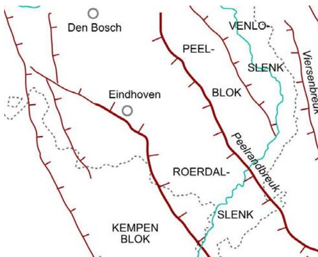
Figuur 4.6. Topografie breuklijnsysteem rond Strabrechtse heide. Figure 4.6. System of fault lines near Strabrechtse heide.
