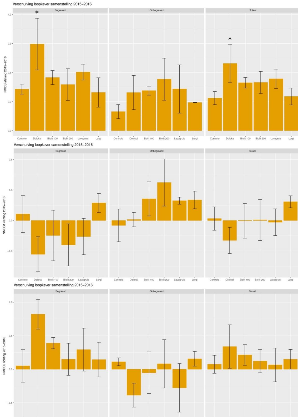
Figuur 9.3. Vergelijking van de verschuiving in soortensamenstelling tussen de verschillende behandelingen, uitgesplitst over begraasde proefvlakken (linker grafieken, n=3 ), onbegraasde proefvlakken (middelste grafieken, n=2 ) en alle proefvlakken samen (rechter grafieken, n=5 ). Boven: verschuiving tussen beide jaren, midden: verschuiving over de 1e as van de NMDS ordinatie. Onder: verschuiving over de 2e as van de NMDS ordinatie. Let op verschillen in schaal tussen de assen. Error bars geven \pm 1 S.E. weer. *: significant verschillend ten opzichte van controle.
