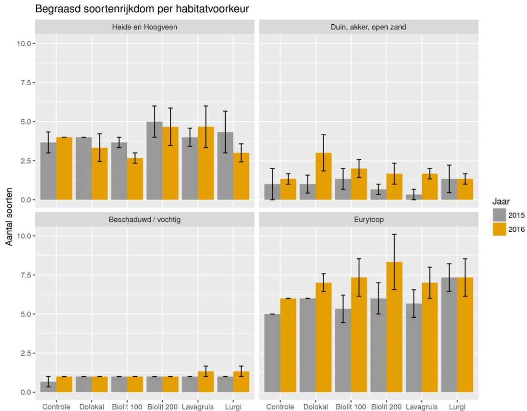
Figuur 9.13. Gemiddelde soortenrijkdom van loopkevers verdeeld over habitatvoorkeur in de verschillende behandelingen van enkel de begraasde proefvlakken ( n=3 ), uitgesplitst over beide bemonsteringsjaren. Error bars geven \pm 1 S.E. weer. *: significant verschillend ten opzichte van controle.
