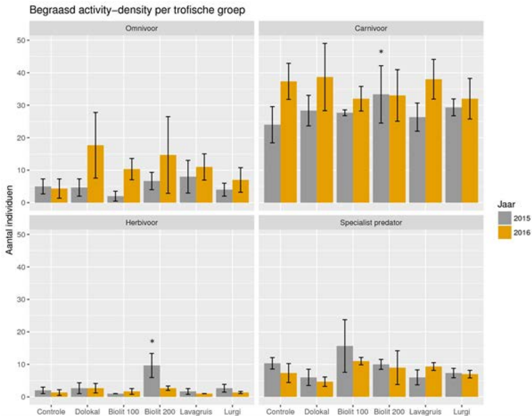
Figuur 9.10. Gemiddelde activity-density van loopkevers verdeeld over trofische groepen in de verschillende behandelingen van enkel de begraasde proefvlakken ( n=3 ), uitgesplitst over beide bemonsteringsjaren. Error bars geven \pm 1 S.E. weer. *: significant verschillend ten opzichte van controle.
