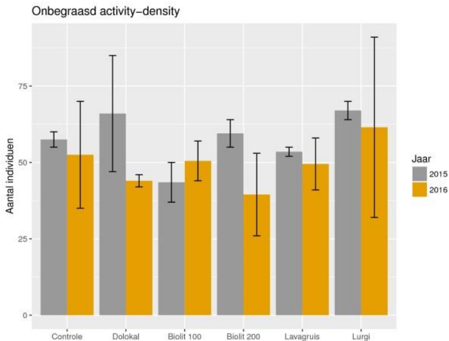
Figuur B6.4. Gemiddelde activity-density van alle loopkevers in de behandelingen van enkel de onbegraasde proefvlakken (n=2), uitgesplitst over beide bemonsteringsjaren. Error bars geven \pm 1 S.E. weer.
