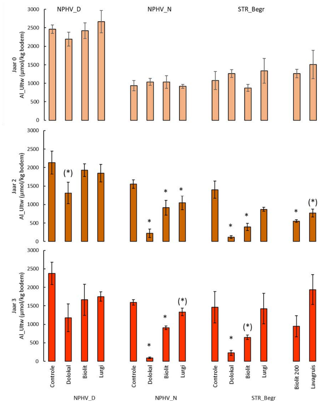
Figuur 5.6. Uitwisselbare concentratie aluminium ( \bar{x} \pm standaard fout, in \mu\text{mol/kg} bodem) in de nulmeting (jaar 0), na twee en na drie effectjaren in de droge proef in het NP de Hoge Veluwe (NPHV_D, links, n=5 ), de natte proeflocatie in het NP De Hoge Veluwe (NPHV_N, midden, n=5 ) en in de begraasde proefvlakken in de droge heide op Strabrecht (STR_Begr, rechts, n=3 ). * = significant verschil ( p < 0,05 ) en (*) = trend ( 0,05 < p < 0,1 ) t.o.v. controle-behandeling binnen hetzelfde jaar.
