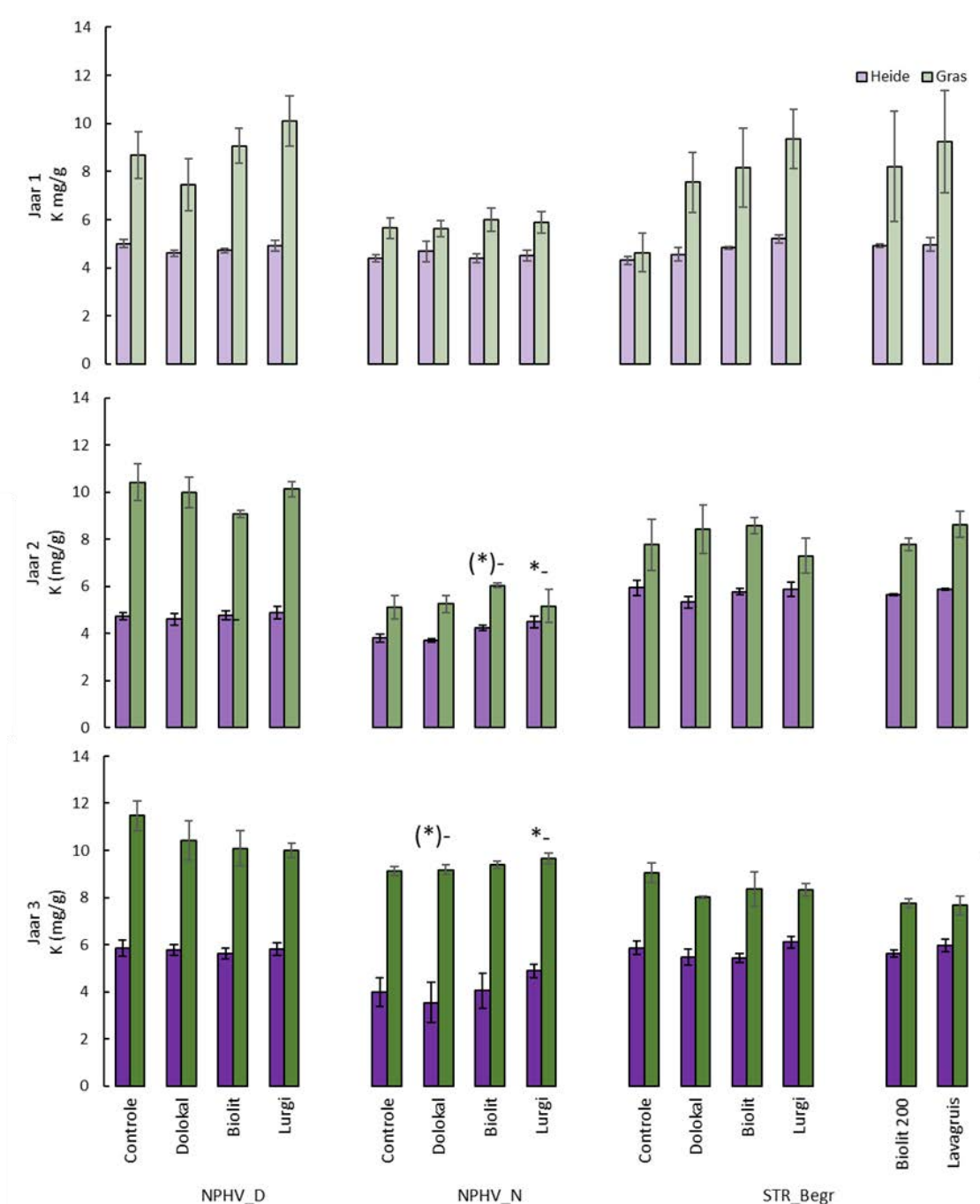
Figuur 6.3. K-concentratie in mg/g droog gewicht gemeten in struikheide (paars), Bochtige smeie (groen) in het NP de Hoge Veluwe (NPHV_D, links, n=5), Dopheide (paars) en Pijpenstrootje (groen) in de natte heide op de Veluwe (NPHV_N, n=5, midden) en Struikheide (paars) en Bochtige smeie (groen) in de begraasde droge heide proefvlakken op Strabrecht (STR_B, rechts, n=3). \bar{x} \pm standaardfout. * =significant verschil ( p < 0,05 ) en (*) =trend ( 0,05 < p < 0,1 ) t.o.v. controle-behandeling binnen hetzelfde jaar. - =geen verschil.
