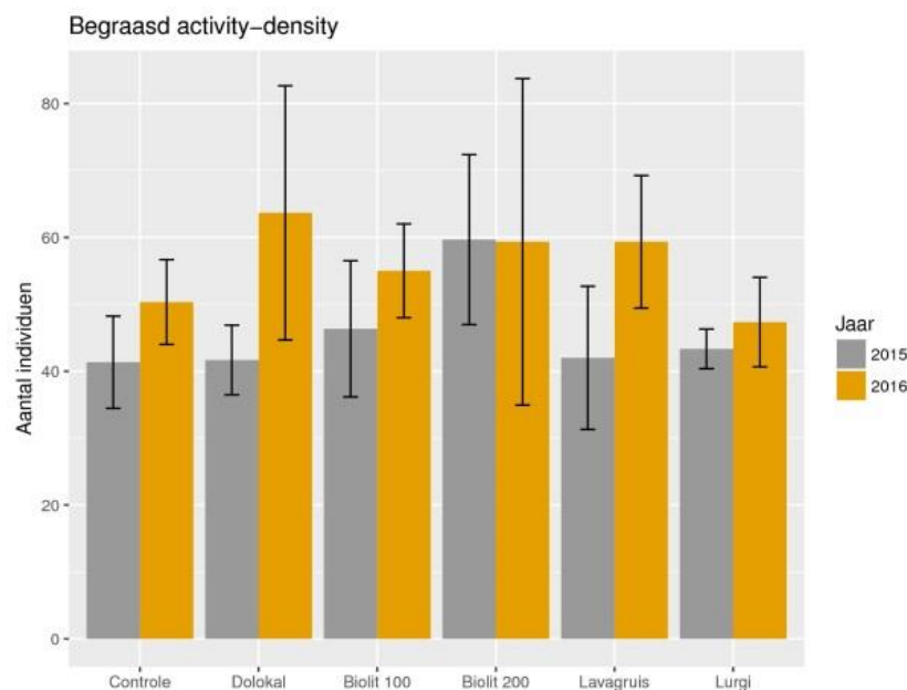
Figuur 9.8. Gemiddelde activity-density van alle loopkevers in de behandelingen van enkel de begraasde proefvlakken ( n=3 ), uitgesplitst over beide bemonsteringsjaren. Error bars geven \pm 1 S.E. weer.
